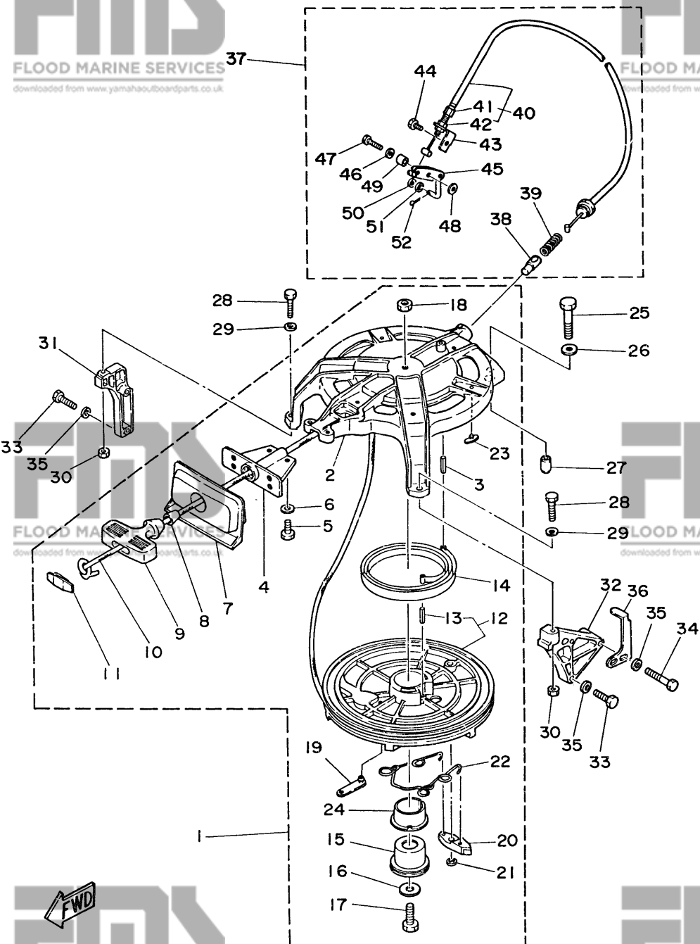
Fig. 4 STARTER
