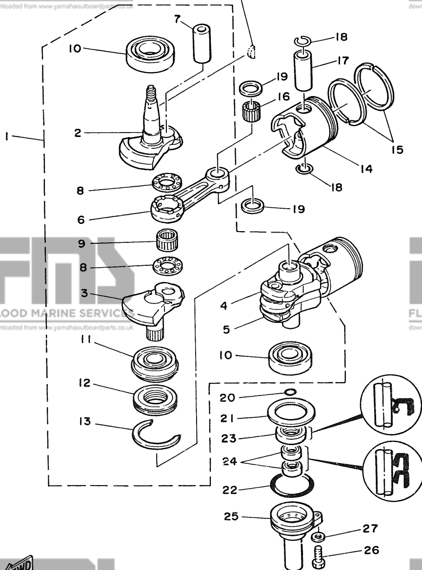
Fig.14, Ref.No.22
