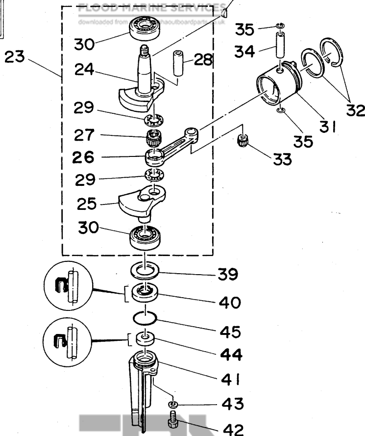
Fig.8, Ref.No.21
