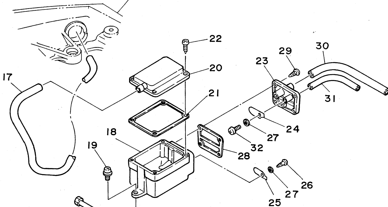
Fig.10, Ref.No.1
