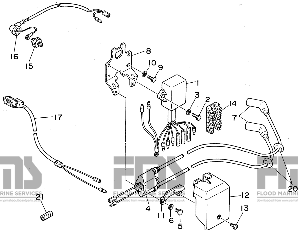
Fig.10, Ref.No.1
