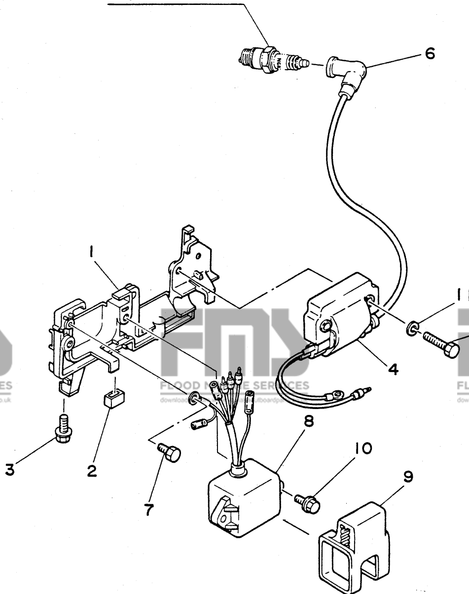
Fig.1, Ref.No.46
