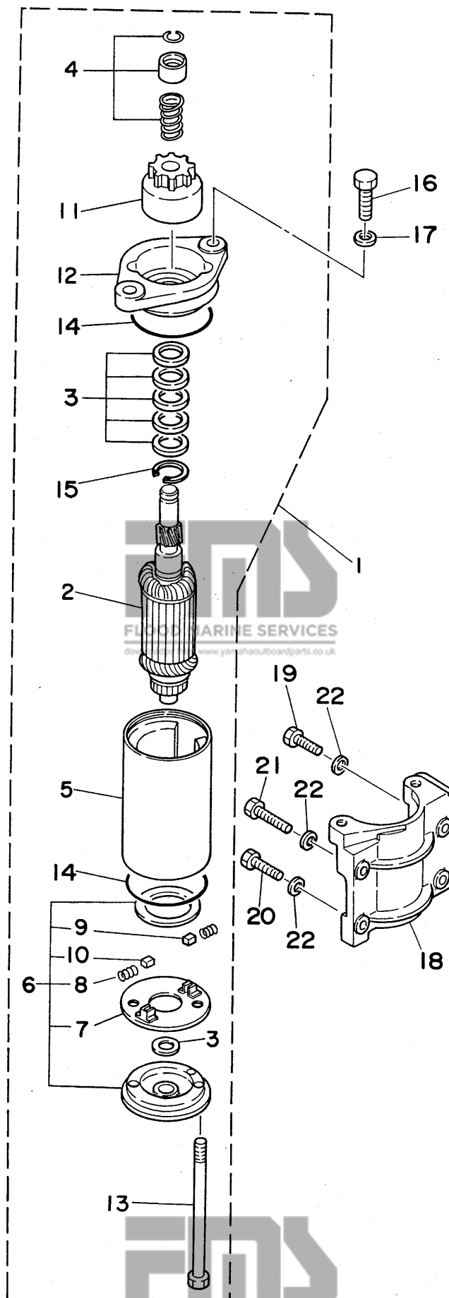
Fig. 15 ELECTRIC MOTOR (9.9DE/15DE MODEL)
