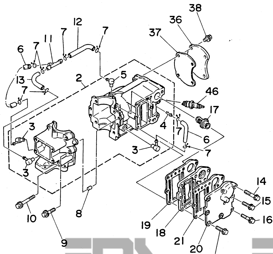
Fig.8, Ref.No.21
