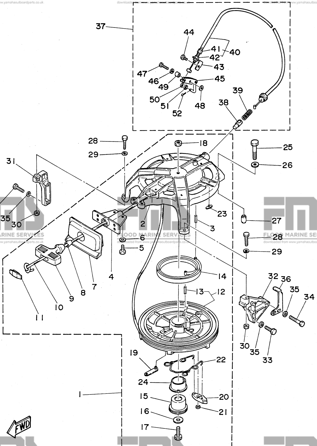
Fig. 4 STARTER
