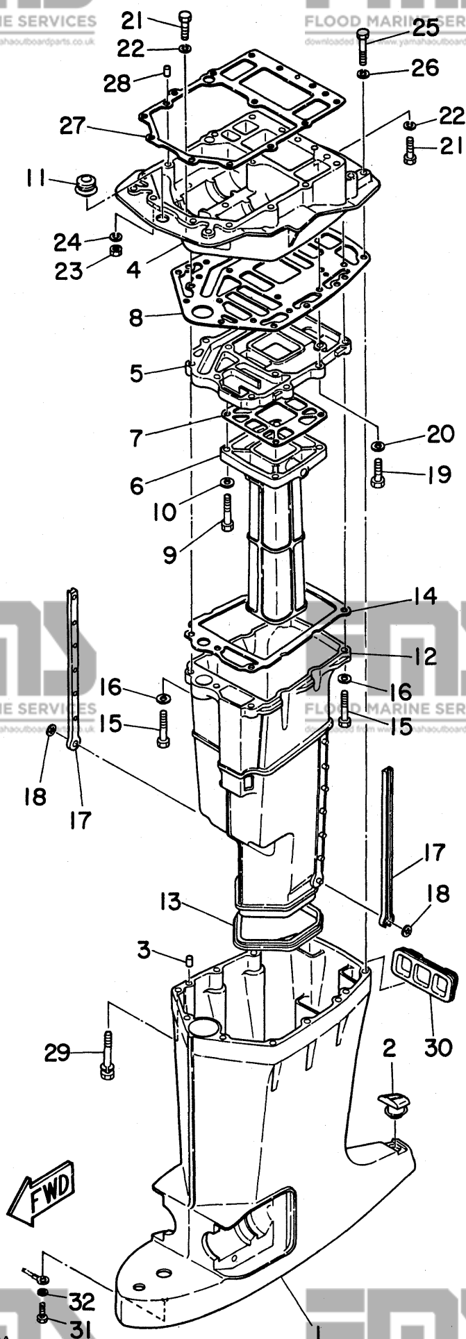
Fig. 12 UPPER CASING
