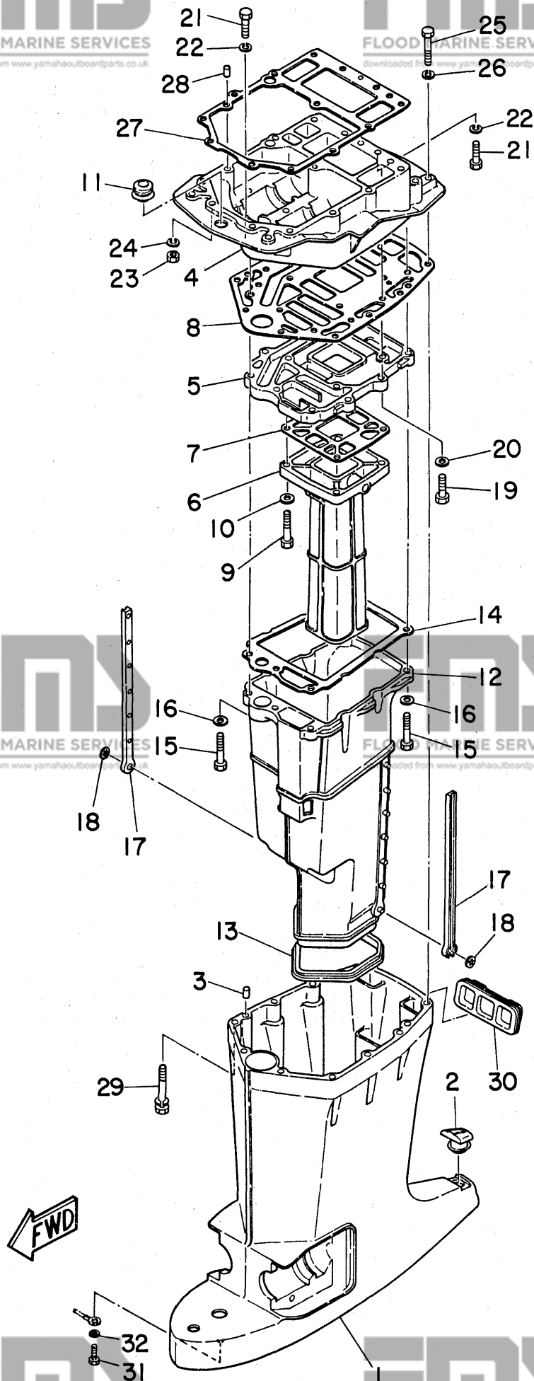
Fig. 1 2 UPPER CASING
