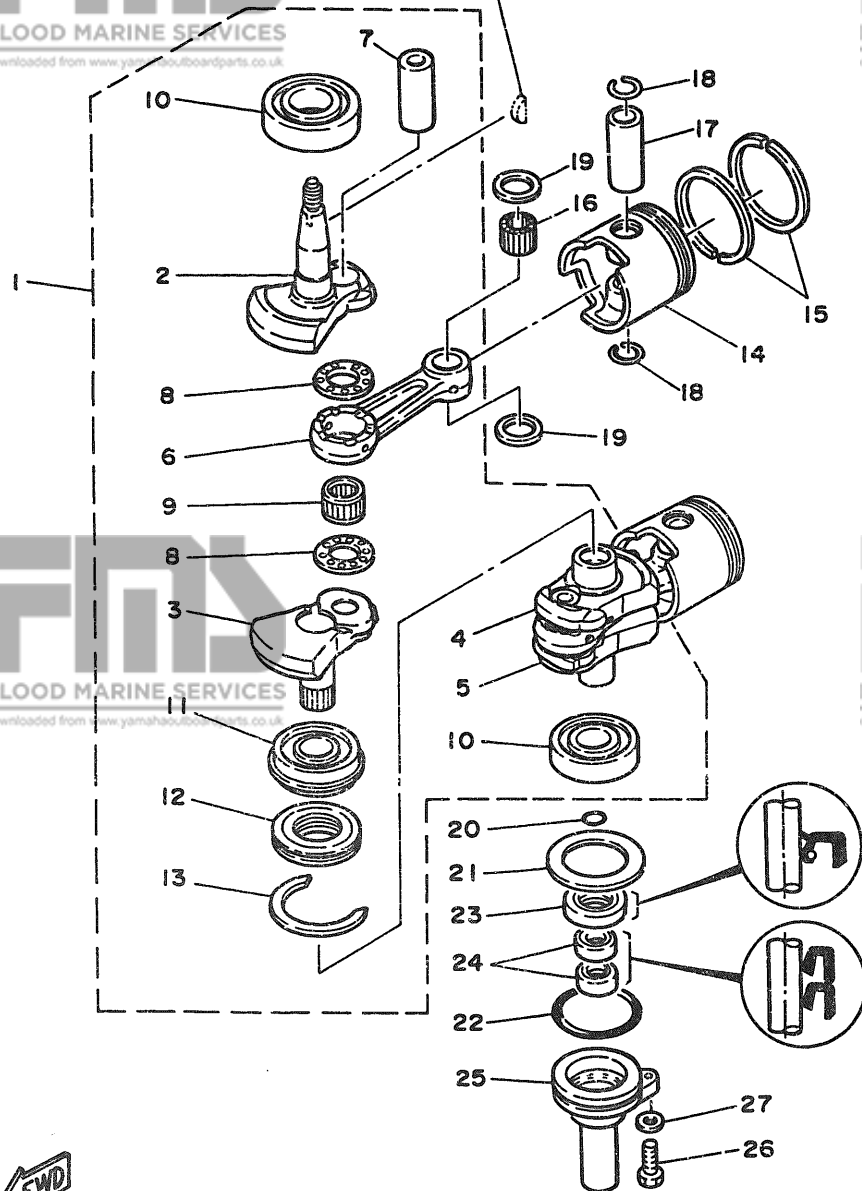
Fig.14, Ref.No.23
