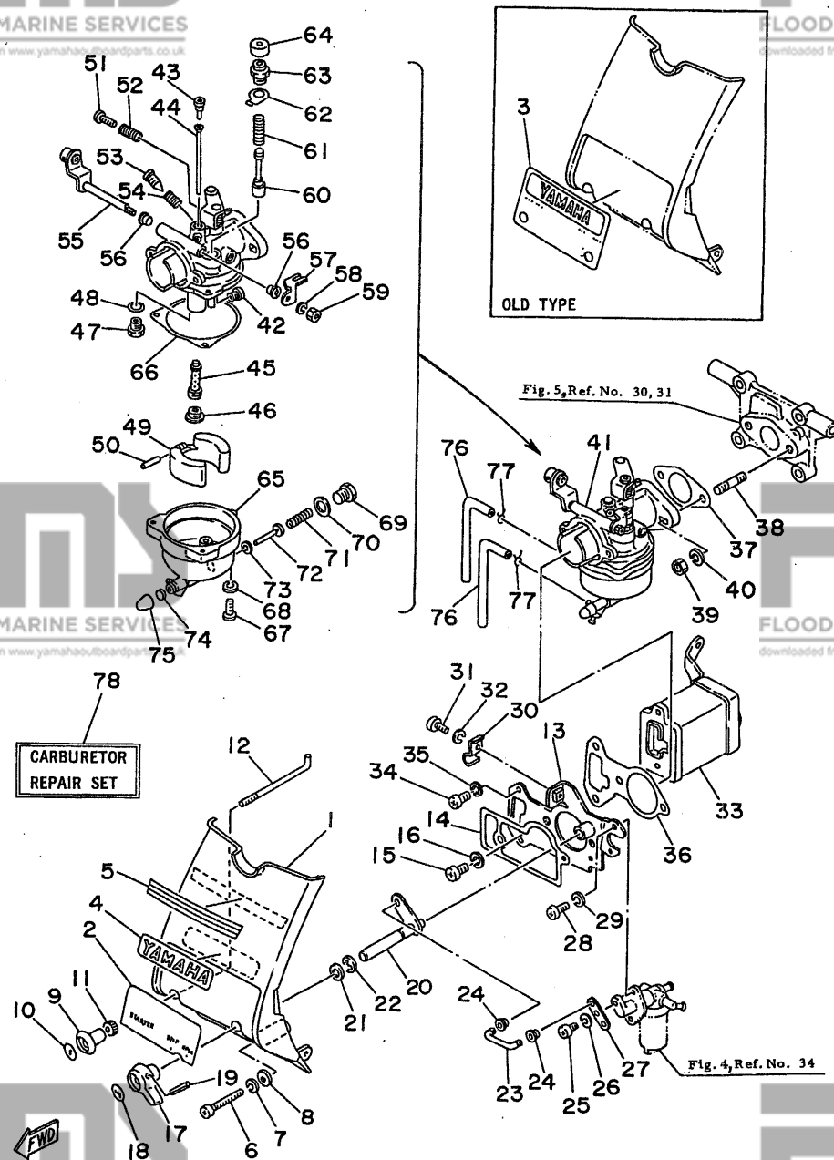
Fig. 6 INTAKE-1979
