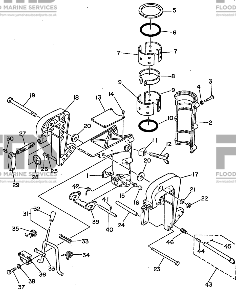
Fig. 9 BRACKET-1979
